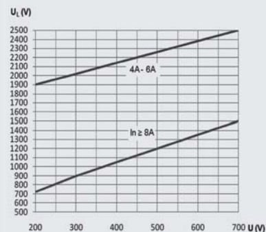
Tensión de Arco ( U_L )
